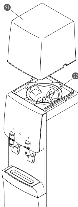
ボトルカバー
